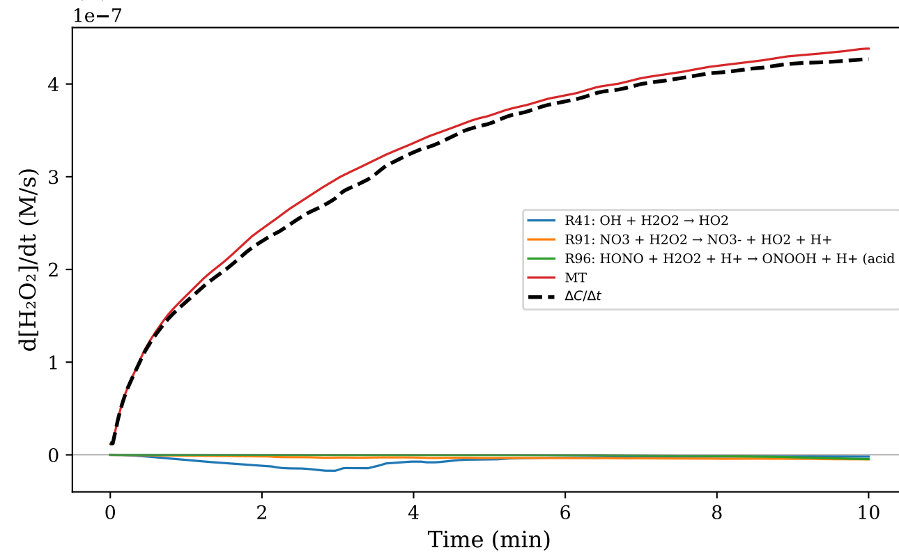
(d) \text{H}_2\text{O}_2
